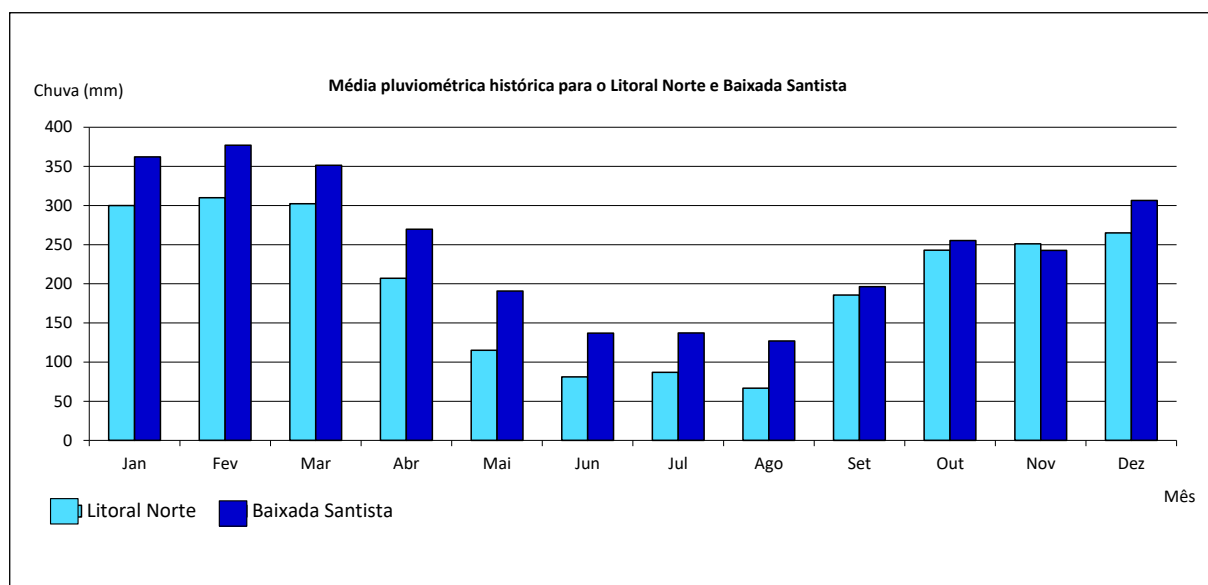
Gráfico 1 – Médias pluviométricas mensais históricas 2
