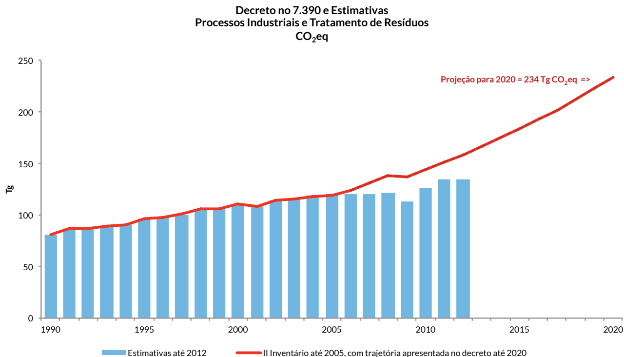
Figura XV – Estimativas de emissão, II Inventário brasileiro e trajetória de emissão para os setores Processos Industriais e Tratamento de Resíduos.
