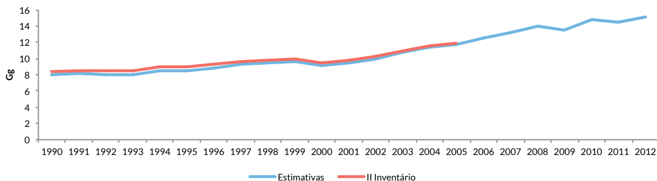
Figura 1.5 Emissões de N 2 O da queima de combustíveis fósseis – setor Energia
