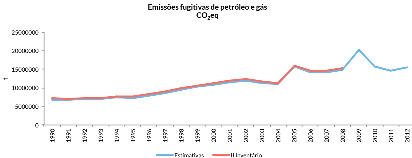
Figura 1.8 Emissões CO 2 eq fugitivas de petróleo e gás, comparação II Inventário e Estimativas, para o setor Energia
