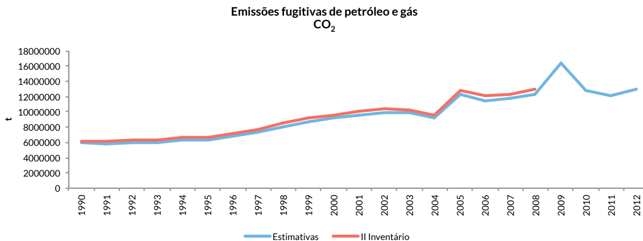
Figura 1.9 Emissões de CO 2 fugitivas de petróleo e gás, comparação II Inventário e Estimativas, para o setor Energia
