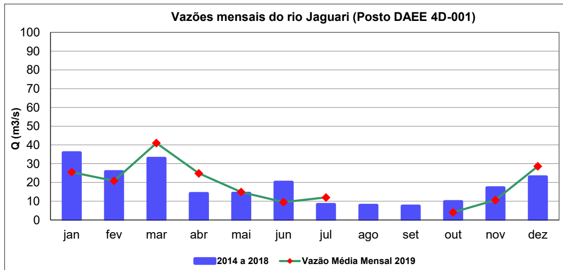
Gráfico 3 – Vazões médias mensais de 2019 e dos últimos 5 anos, no Ponto JAGR 02800.
