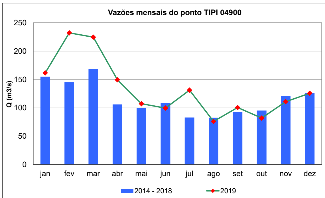
Gráfico 7 – Vazões médias mensais de 2019 e dos últimos 5 anos, no Ponto TIPI 04900.
