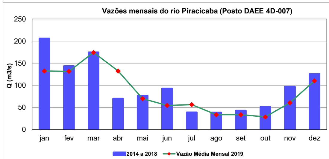
Gráfico 5 – Vazões médias mensais de 2019 e dos últimos 5 anos, no Ponto PCAB 02800.
