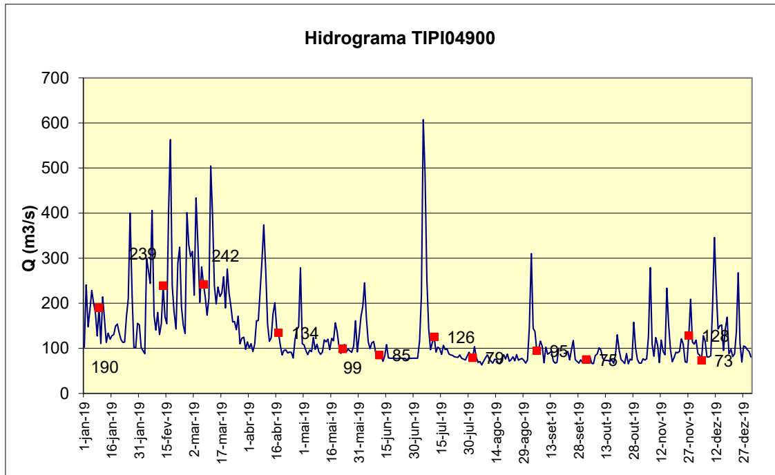
Gráfico 8 – Vazões médias diárias e vazões nas datas de coleta em 2019, no Ponto TIPI 04900.
