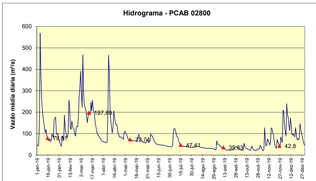
Gráfico 6 – Vazões médias diárias e vazões nas datas de coleta em 2019, no Ponto PCAB 02800.
