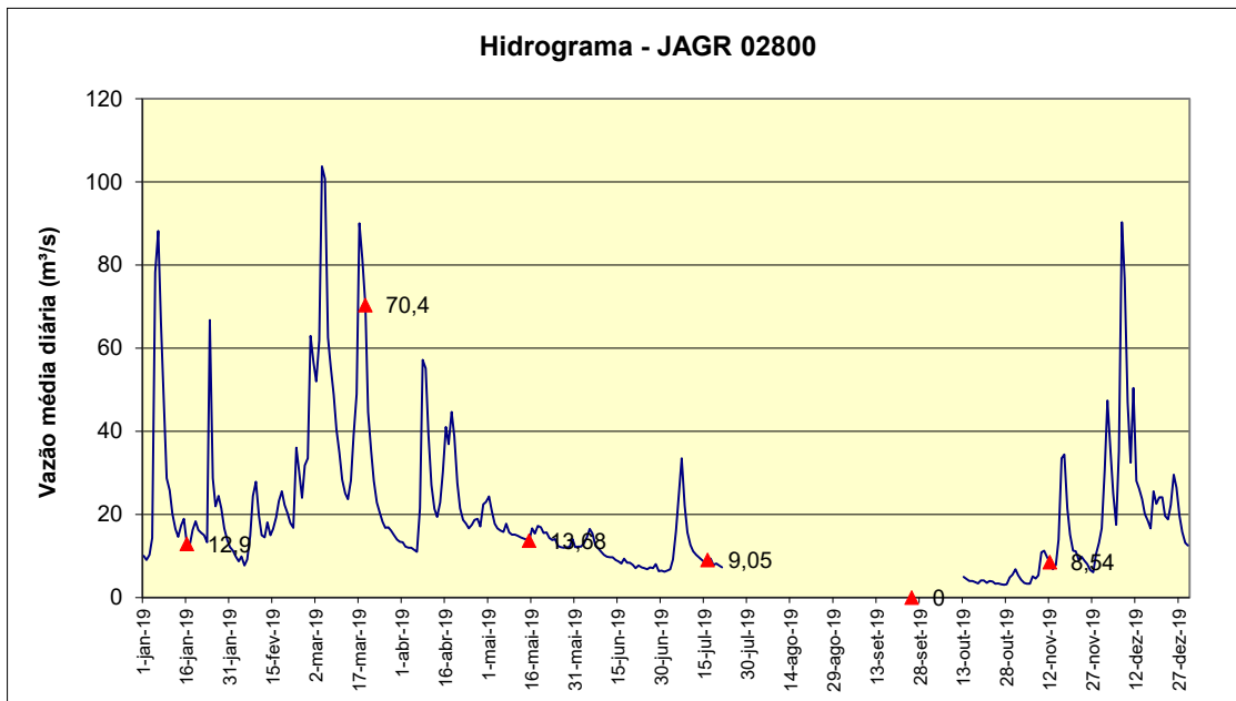
Gráfico 4 – Vazões médias diárias e vazões nas datas de coleta em 2019, no Ponto JAGR 02800.
