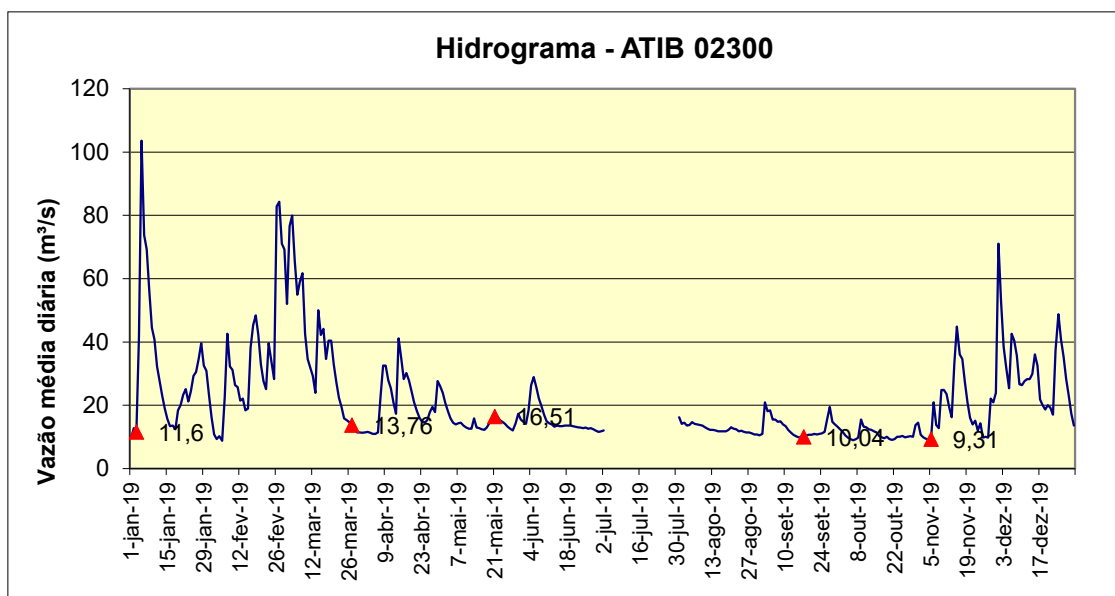
Gráfico 2 – Hidrograma do Posto DAEE 4D-009 e vazões nas datas de coleta do ponto ATIB 02300 – 2019.
