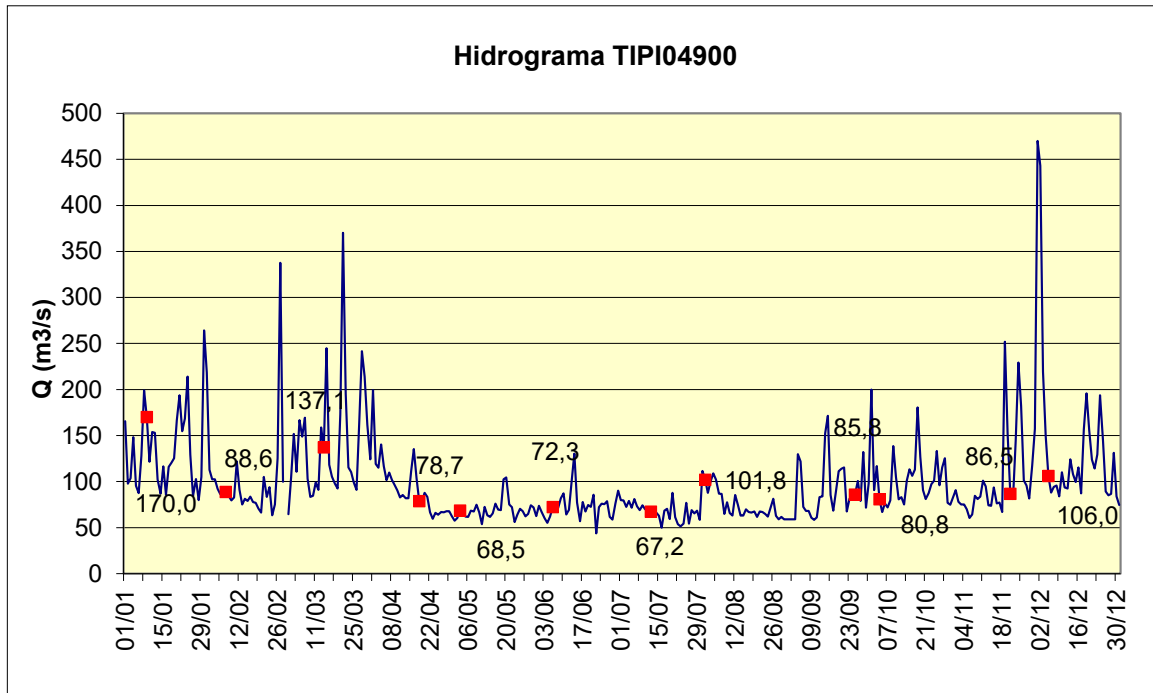
Gráfico 8 – Vazões médias diárias e vazões nas datas de coleta em 2017, no Ponto TIPI 04900.
