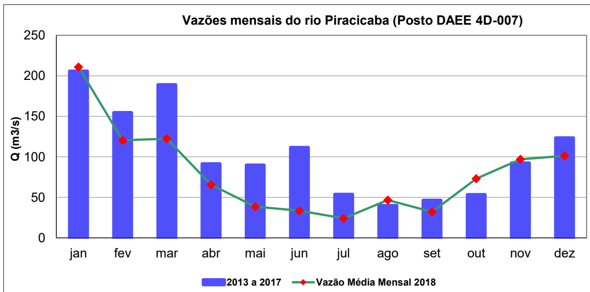
Gráfico 5 – Vazões médias mensais de 2018 e dos últimos 5 anos, no Ponto PCAB 02800.
