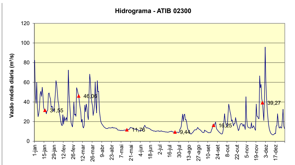
Gráfico 2 – Hidrograma do Posto DAEE 4D-009 e vazões nas datas de coleta do ponto ATIB 02300 - 2018.
