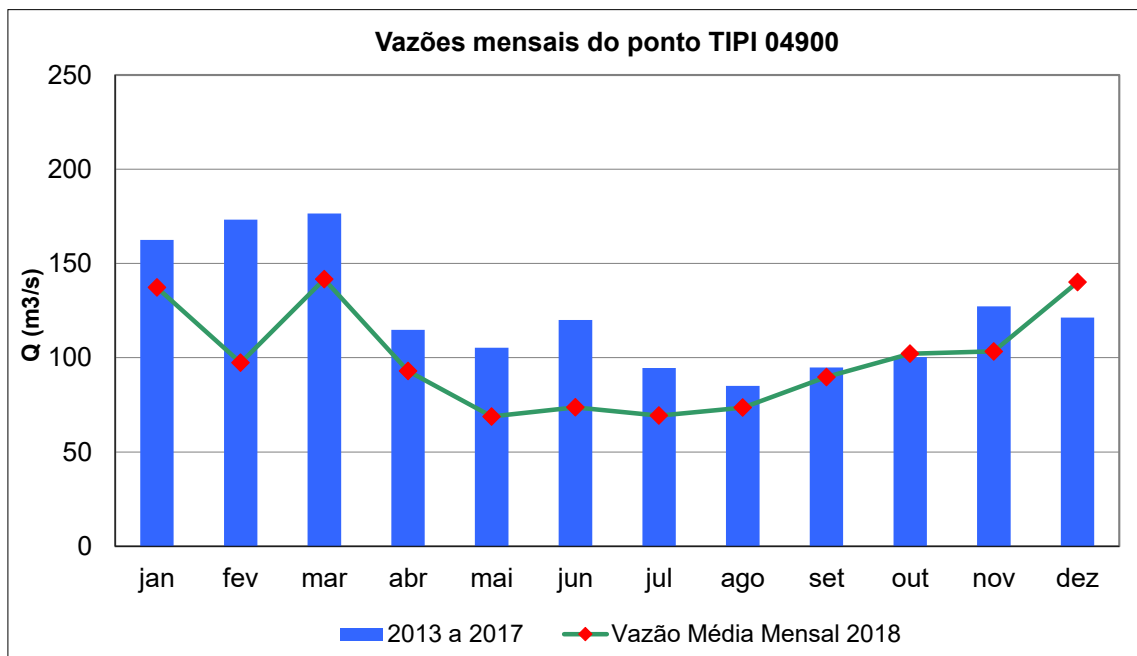
Gráfico 7 – Vazões médias mensais de 2018 e dos últimos 5 anos, no Ponto TIPI 04900.
