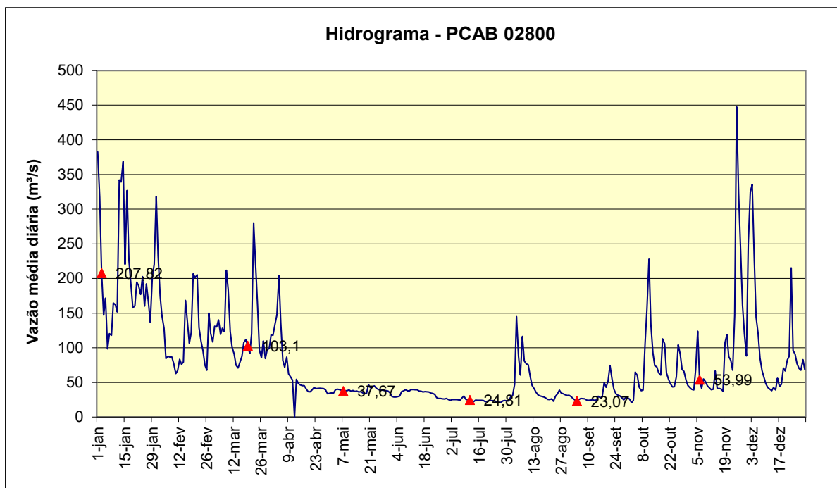
Gráfico 6 – Vazões médias diárias e vazões nas datas de coleta em 2018, no Ponto PCAB 02800.
