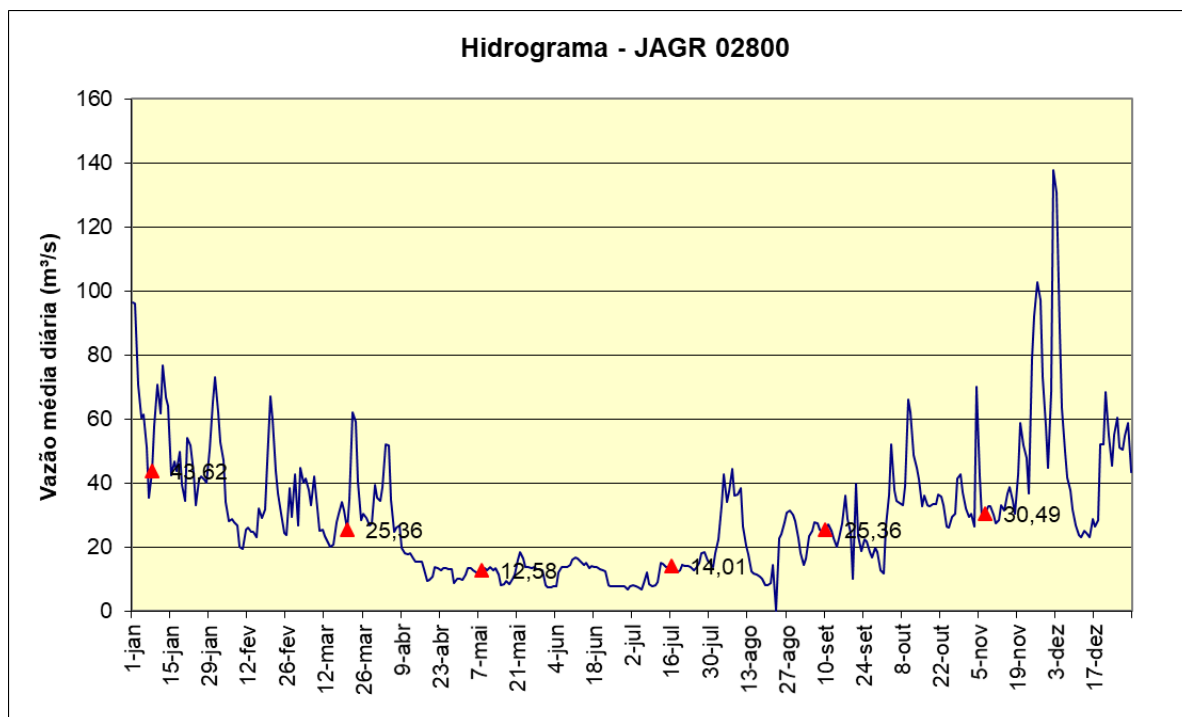
Gráfico 4 – Vazões médias diárias e vazões nas datas de coleta em 2018, no Ponto JAGR 02800.
