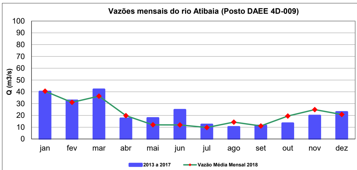
Gráfico 1 – Vazões médias mensais de 2018 e dos últimos 5 anos, no Ponto ATIB 02300.
