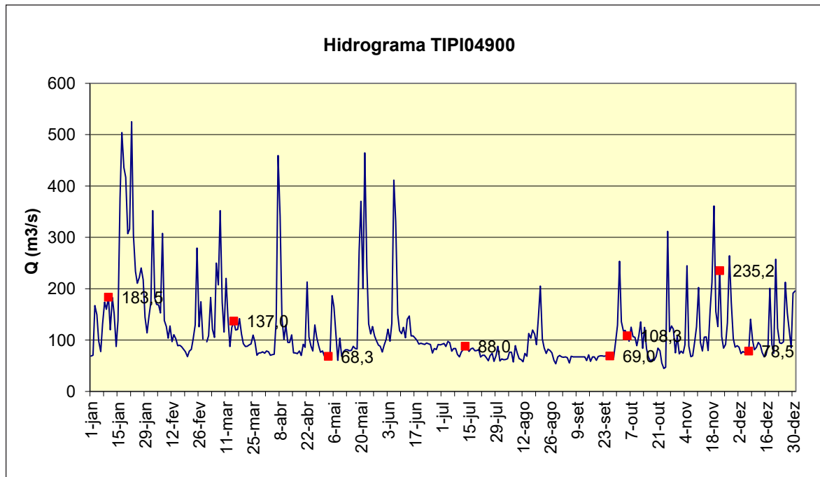
Gráfico 8 – Vazões médias diárias e vazões nas datas de coleta em 2017, no Ponto TIPI 04900.
