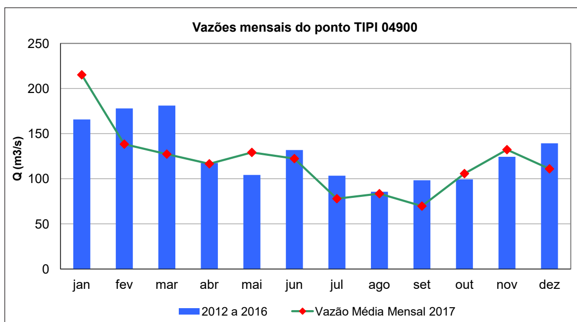
Gráfico 7 – Vazões médias mensais de 2017 e dos últimos 5 anos, no Ponto TIPI 04900.
