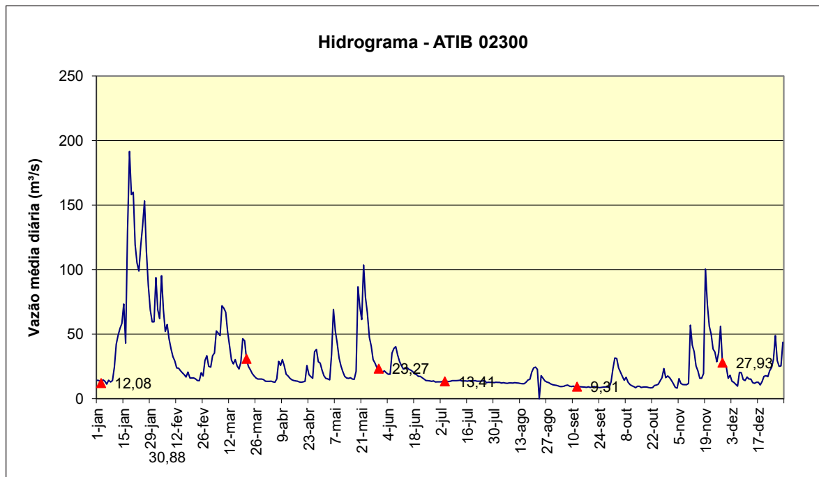
Gráfico 2 – Hidrograma do Posto DAEE 4D-009 e vazões nas datas de coleta do ponto ATIB 02300 - 2017.
