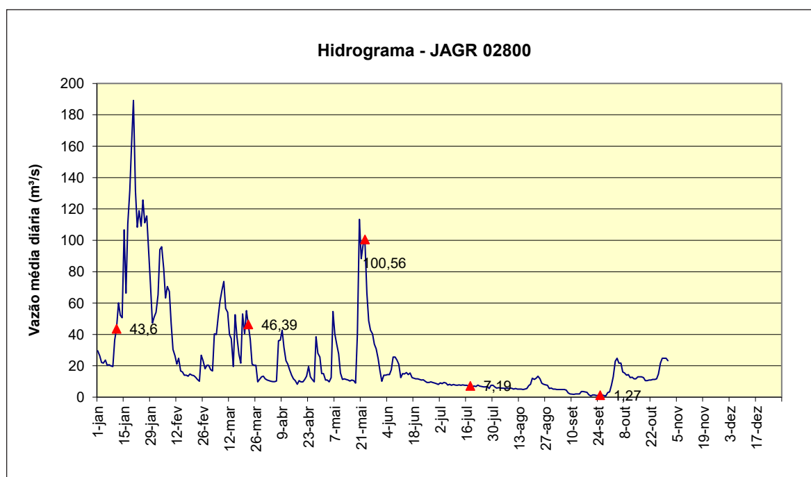
Gráfico 4 – Vazões médias diárias e vazões nas datas de coleta em 2017, no Ponto JAGR 02800.
