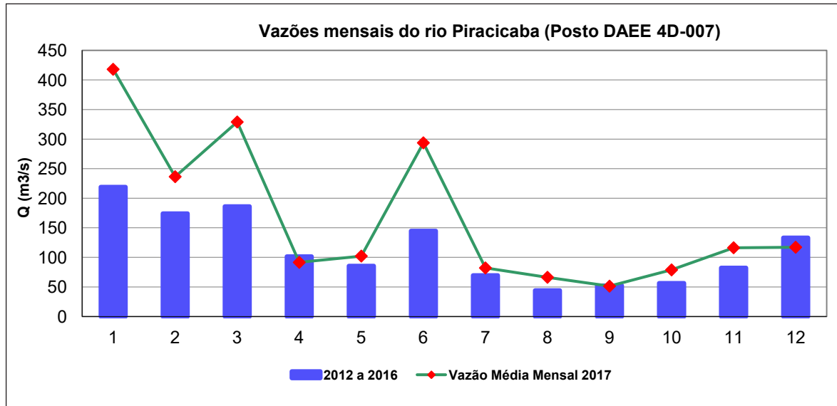
Gráfico 5 – Vazões médias mensais de 2017 e dos últimos 5 anos, no Ponto PCAB 02800.
