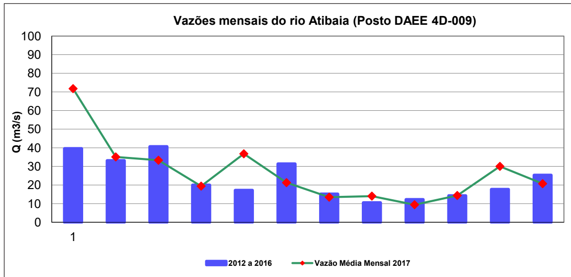
Gráfico 1 – Vazões médias mensais de 2017 e dos últimos 5 anos, no Ponto ATIB 02300.
