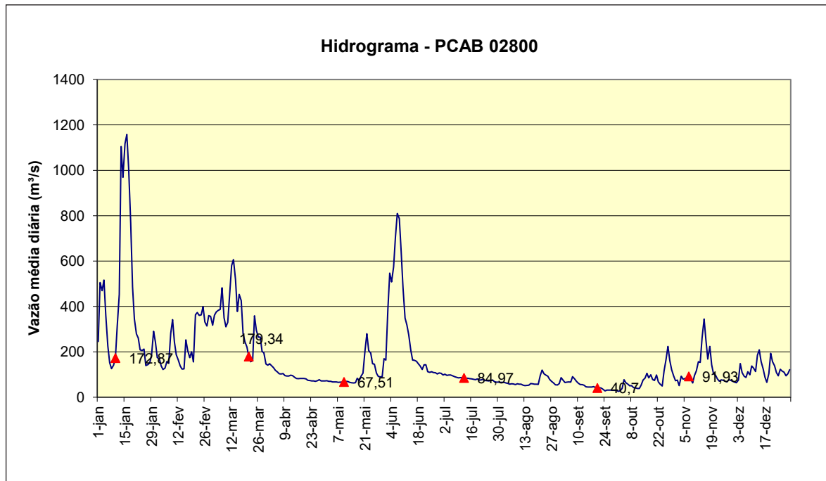
Gráfico 6 – Vazões médias diárias e vazões nas datas de coleta em 2017, no Ponto PCAB 02800.
